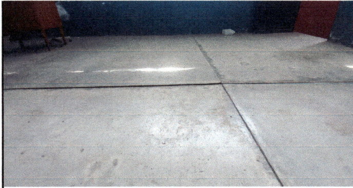
Foto 7: Aula 2 del módulo 3. Tarta de concreto en pésimas condiciones con hundimiento, que necesita ser reemplazado.
