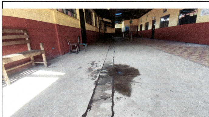
Foto 2: Tubería de aguas pluviales colapsado frente módulo 2, necesita remoción y sustitución por tubería PVC 8".
